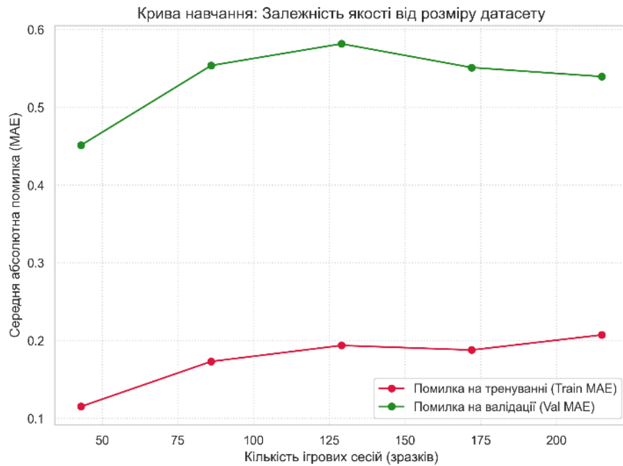
Рис. 3.12 Крива навчання багатошарового перцептронну
